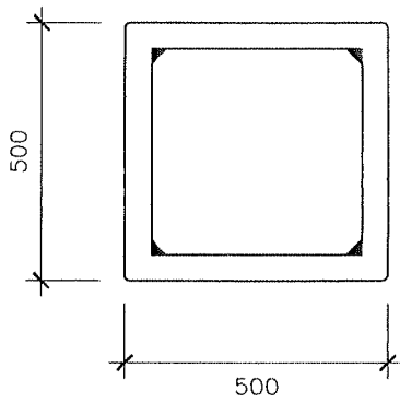
PLAN P.B 24 SCALE: 1:15
